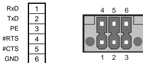
6pol. Combicon-Stecker COM1
